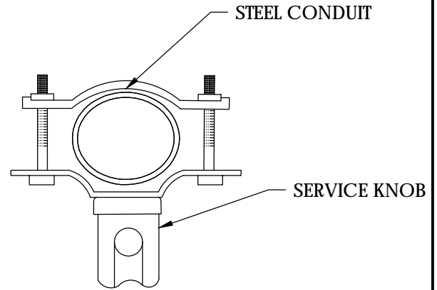
PIPE RISER
